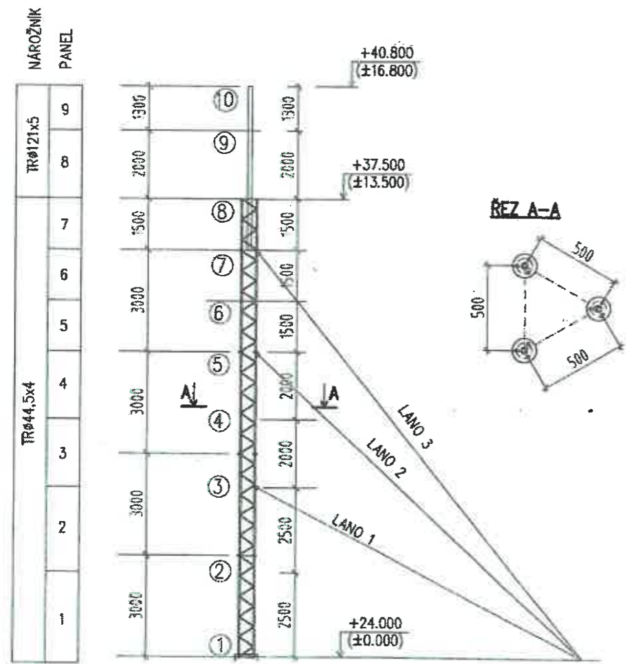
Obr. 4.1 Schéma konstrukce
